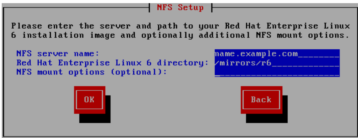
그림 15.10. NFS 설정 대화 상자
