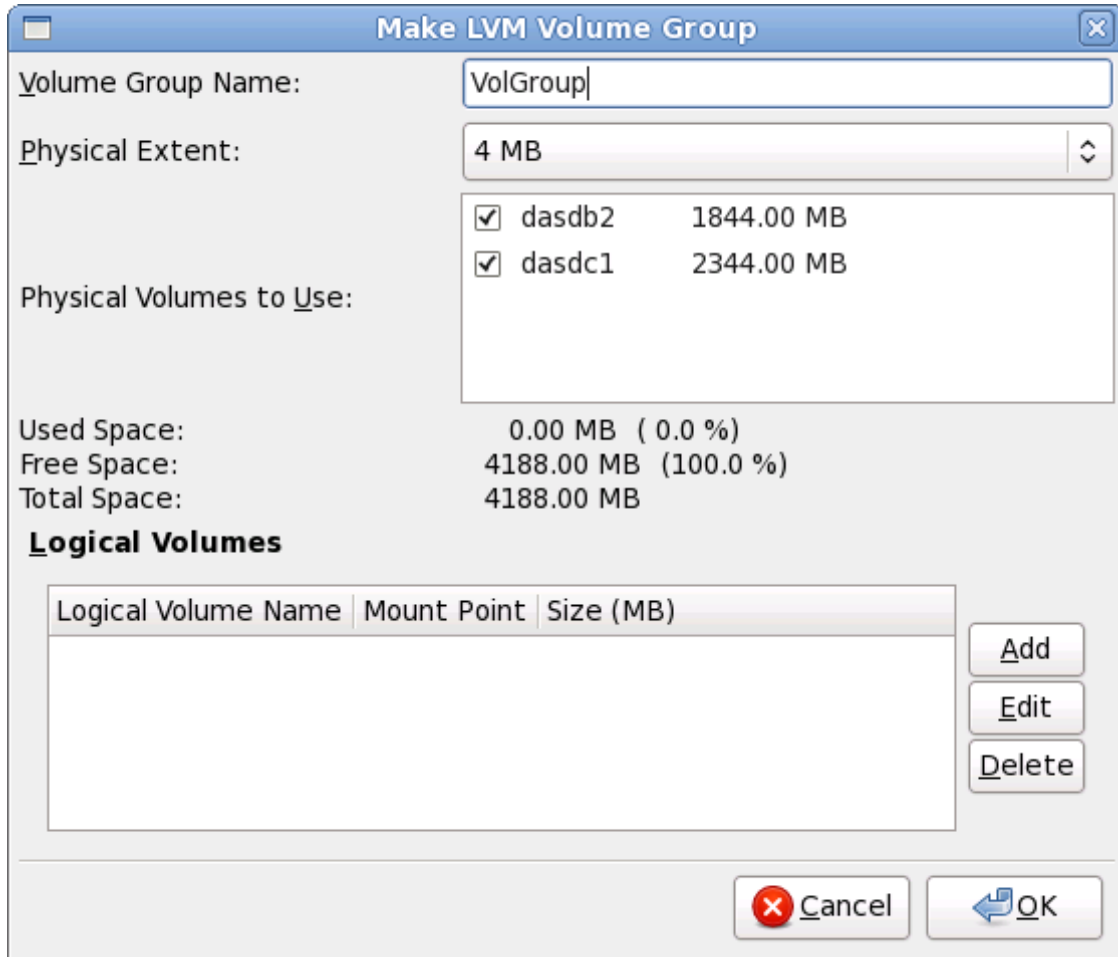
그림 23.43. 볼륨 그룹 만들기
