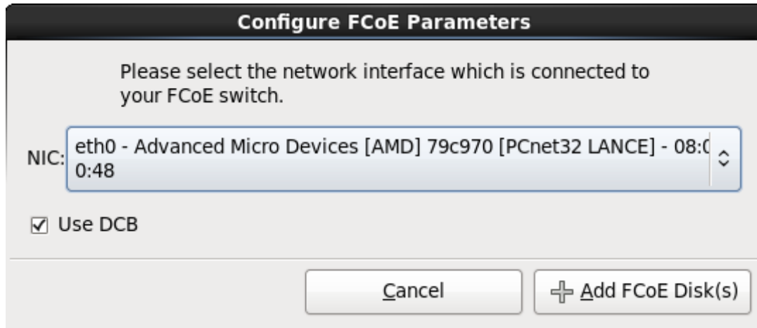
그림 9.22. FCoE 파라미터 설정
