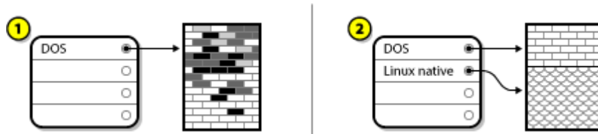
그림 A.10. 파괴적으로 재파티션된 디스크 드라이브
