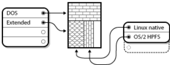
그림 A.7. 확장 파티션을 가진 디스크 드라이브
